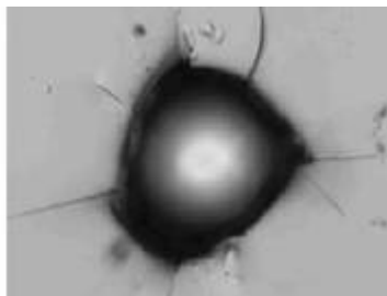
keimende Sporen
